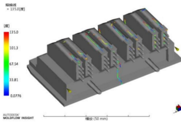
Weld Lines(熔接线)
