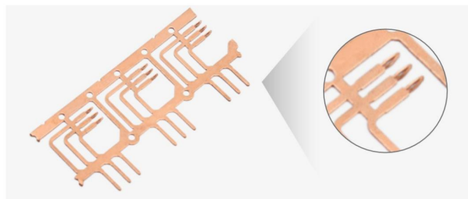
免焊端子系列 Press-Fit Connections
